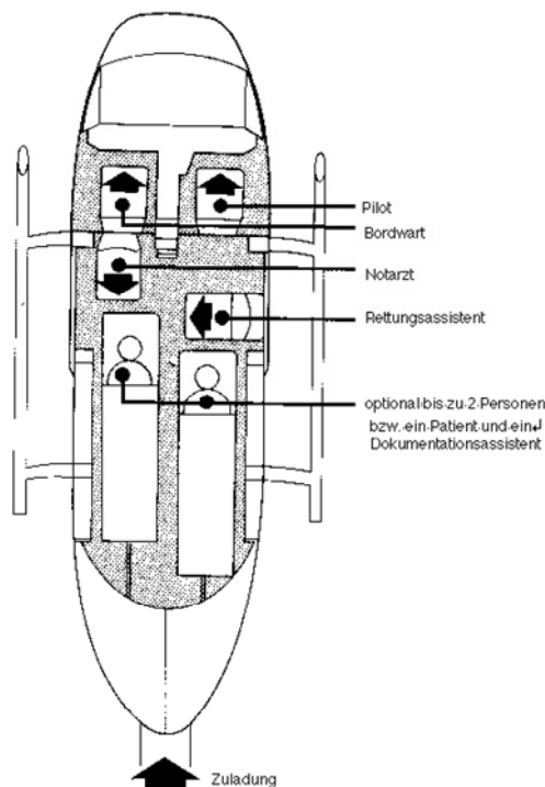
Abbildung 5: Innenraum-Schema der BK 117 [26]
