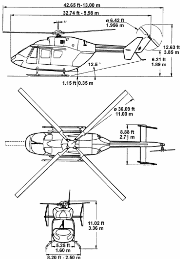
Abbildung 4: Schematische Darstellung der BK 117 [26]
