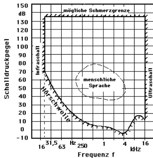
Abb. 2: Die Hörschwelle des menschlichen Ohres in Abhängigkeit von der Frequenz (Schalldruckpegel hier in dB aufgetragen) (Grafik: U. Dietze – Fritz-Süchting-Institut für Maschinenwesen – TU Clausthal).
