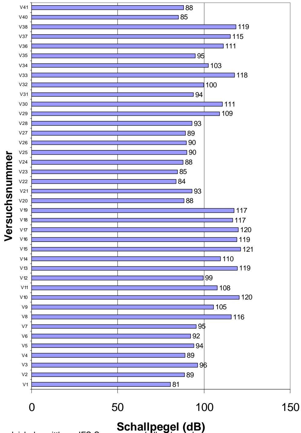
Abb. 9: Vergleich der mittleren IFS-Summenpegel aller Versuche.
