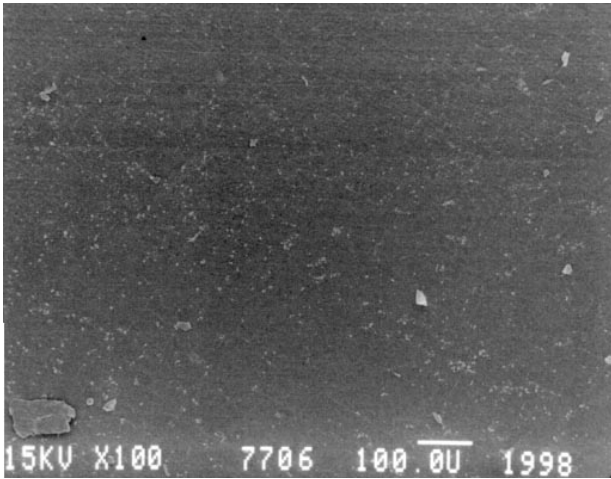
Schlauch Nr. 2 Innenfläche: Ungebrauchter, steriler Schlauch bei 100-facher Vergrößerung
