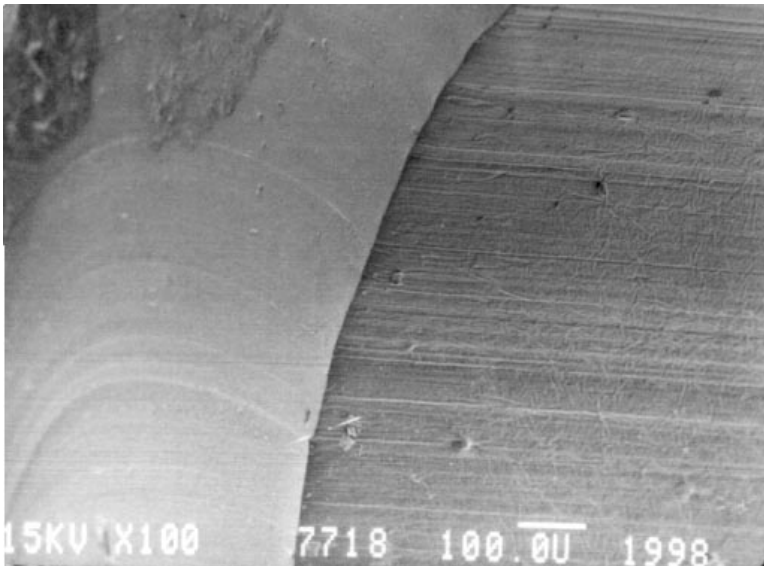
Schlauch Nr. 2: Ungebrauchter, steriler Schlauch bei 100-facher Vergrößerung: Hier ist eine glatte Schnittfläche zu sehen.
