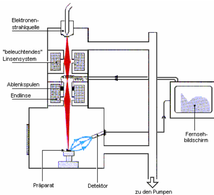
Der optische Weg in einem Rasterelektronenmikroskop
