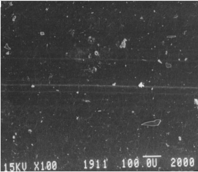
Schlauch Nr. 6 Innenfläche: Einwegsystem bei 100-facher Vergrößerung: Innenfläche intakt
