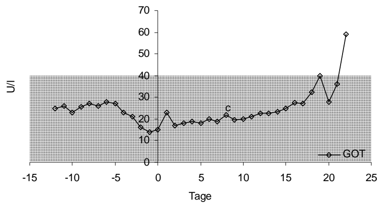
Abb. 4.2.3: Darstellung des Glutamat-Oxalacetat-Transaminaseverlaufes (GOT) in U/l, gemessen über die Zeit, ab Tag -12 vor Transplantation (Tag 0) bis Tag +22 nach Transplantation. Die Datenpunkte repräsentieren dabei den Median, welcher sich aus den GOT- Werten aller gemessenen Patienten für den jeweiligen Tag ergibt. Der Graubereich entspricht dem Normalbereich.
