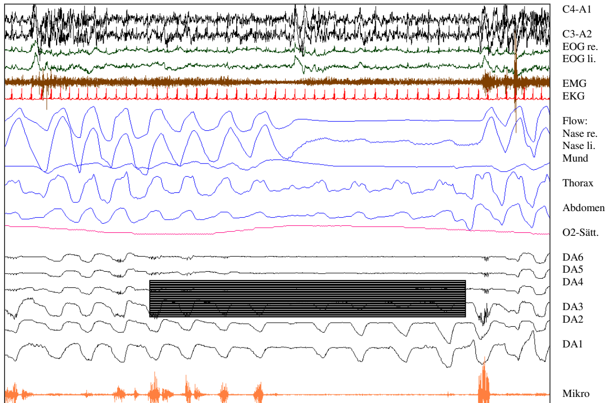
Abb. 18: Retrolinguale Obstruktion.
