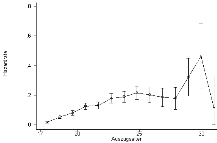
Abbildung 6.2: Hazardrate
