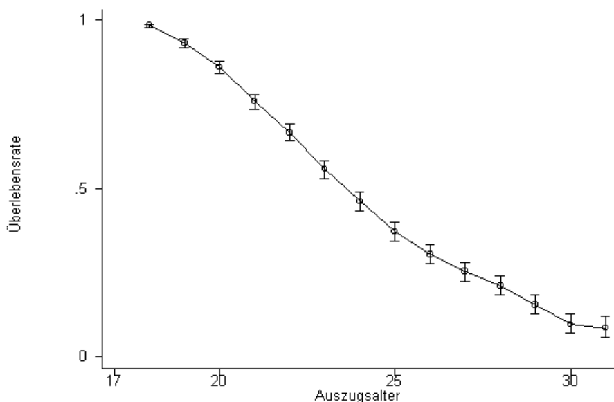
Abbildung 6.1: Überlebensrate
