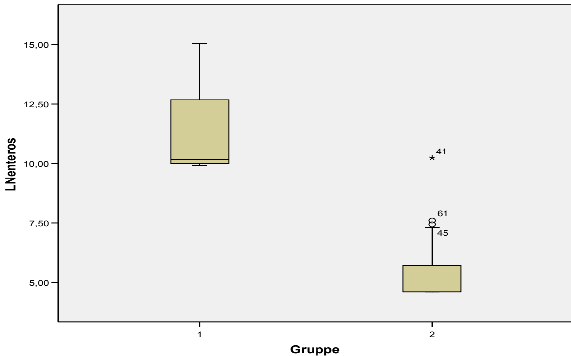
Abb. 4: Boxplot-Diagramm für die Mittelwerte des Parameters Enterobakteriäzen. Es werden die Gruppe I (Ware, die in dem Betrieb weiterverarbeitet wurde) und die Gruppe II (Ware, die in dem Betrieb ausschließlich gelagert wurde) gegenübergestellt
