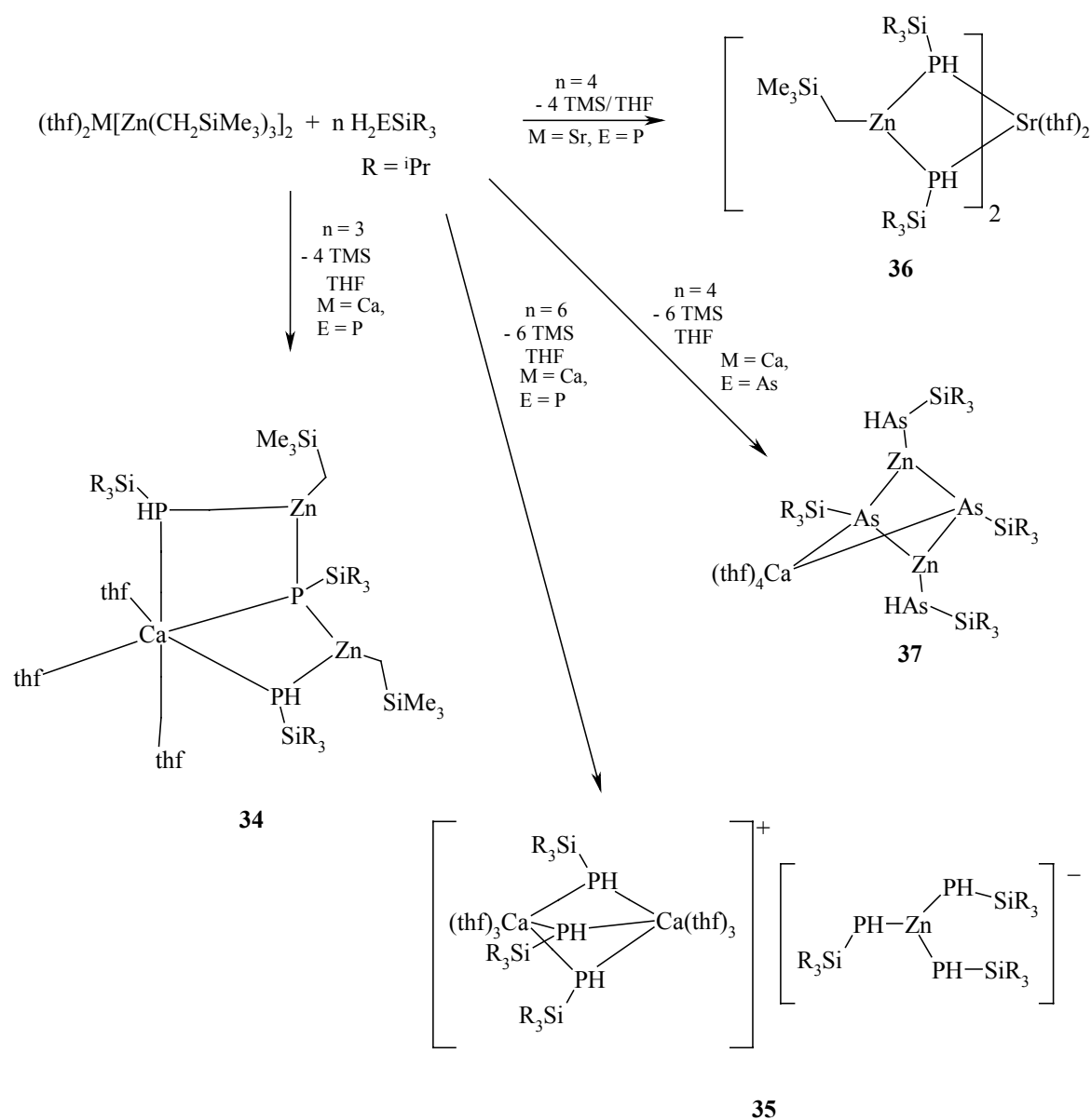
Reaktionsschema 4.6: Umsetzung von Calcium-bis[tris(trimethylsilylmethyl)zinkat] 24 mit primären Silylpentanen.
