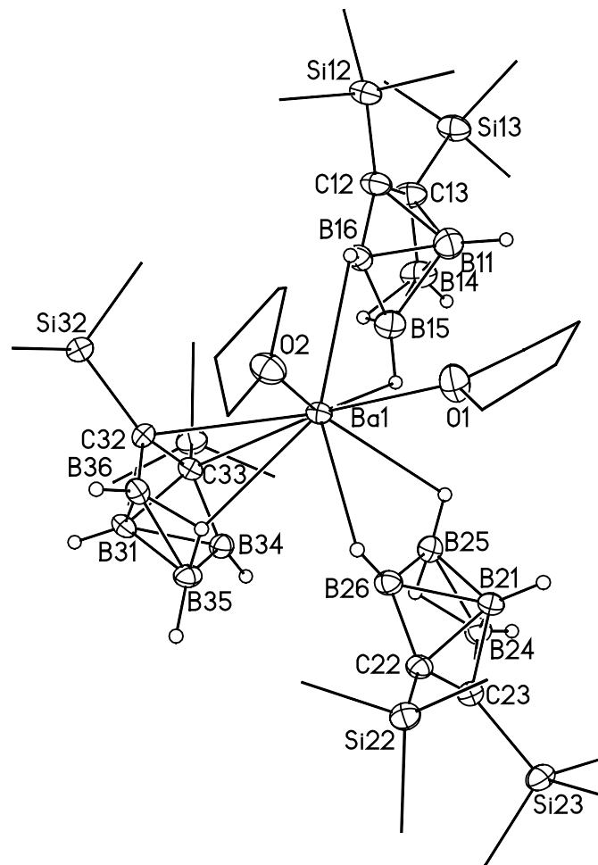
Abbildung 2.25: Die Koordinationssphäre der Bariumatome in dimerem Bis(tetrahydrofuran- O )barium-bis[bis-2,3-(trimethylsilyl)-2,3-dicarba-hexaboranat] 33 . Die Thermal ellipsoide der Schweratome repräsentieren eine Aufenthaltswahrscheinlichkeit von 40%. Die Wasserstoffatome sind mit willkürlichen Radien gezeichnet.
